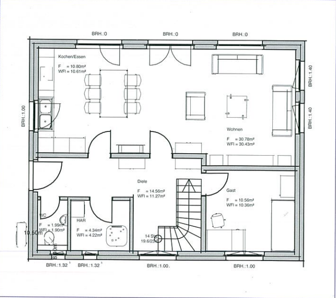
ERDGESCHOSS STADTHAUS TYP 2
