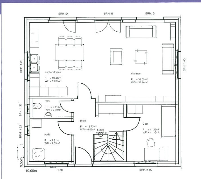
ERDGESCHOSS STADTHAUS TYP 1
