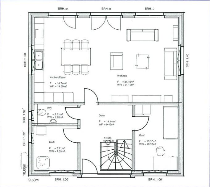
ERDGESCHOSS STADTVILLA TYP 2
