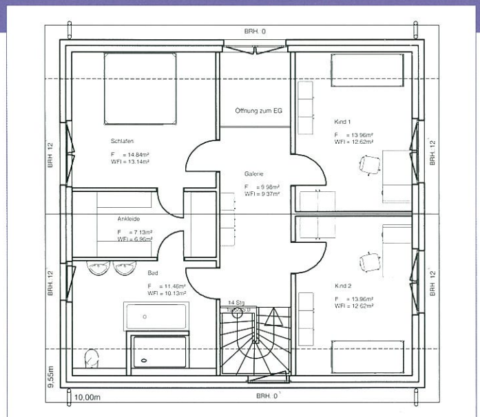
OBERGESCHOSS STADTHAUS TYP 1
