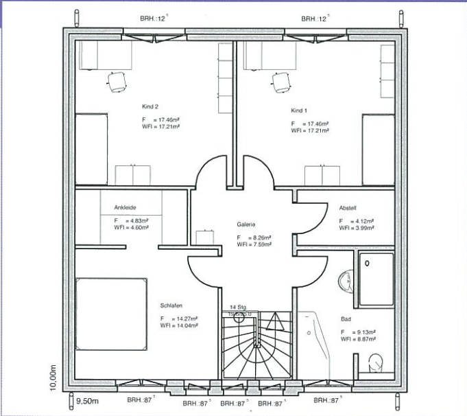
OBERGESCHOSS STADTVILLA TYP 2
