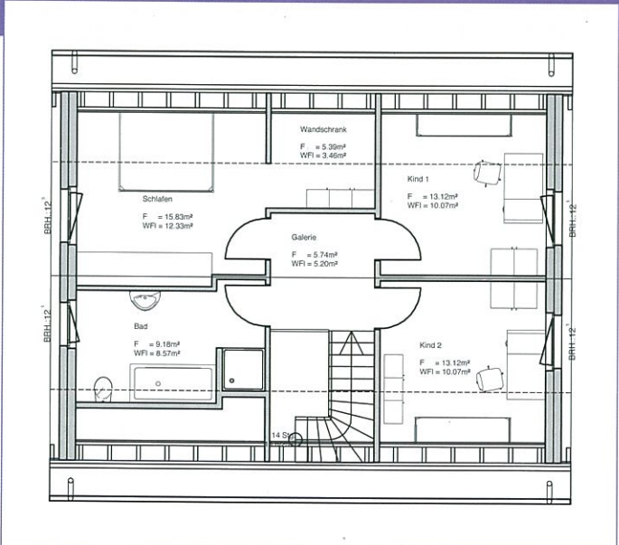
OBERGESCHOSS STADTHAUS TYP 2
