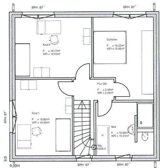
OBERGESCHOSS STADTVILLA TYP 1
